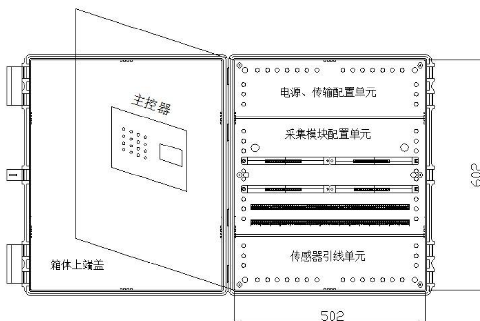
图一 SWN-102 机箱结构示意图
